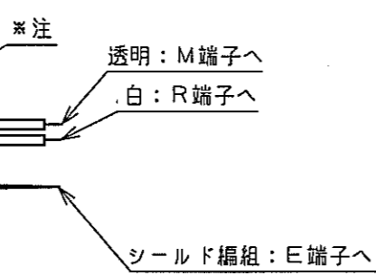
C-2A 中継ケーブル端末処理方法
