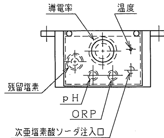
測定セル電極取付位置 A 視図
