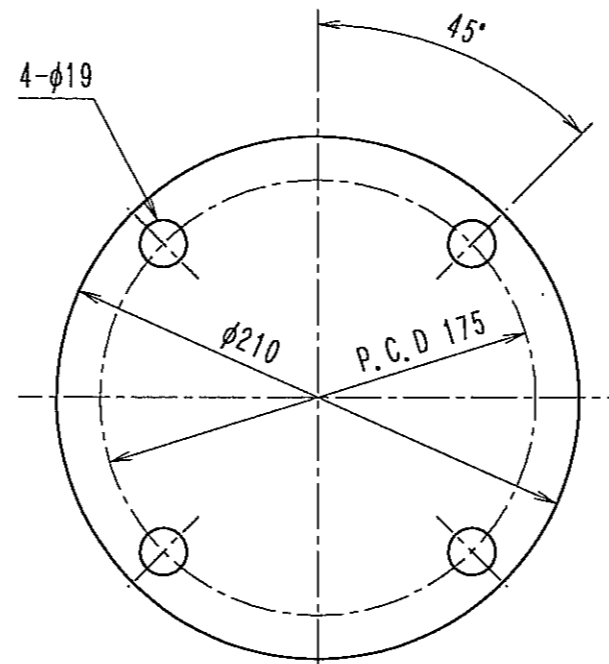
JIS10K 100Aに準用 取付座詳細
