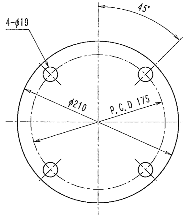
JIS10K 100Aに準用 取付座詳細
