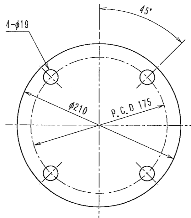
JIS10K 100Aに準用 取付座詳細
