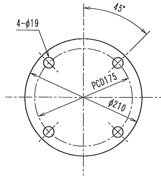
JIS 10K 100Aに準用 取付座詳細
