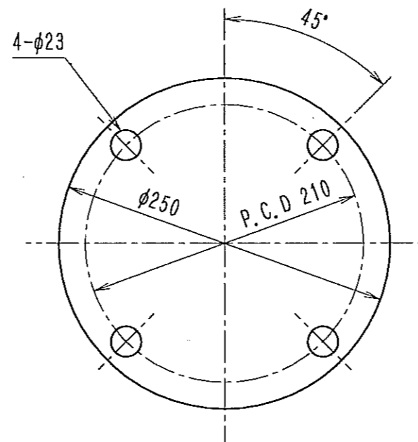
JIS 10K 125Aに準用 取付座詳細
