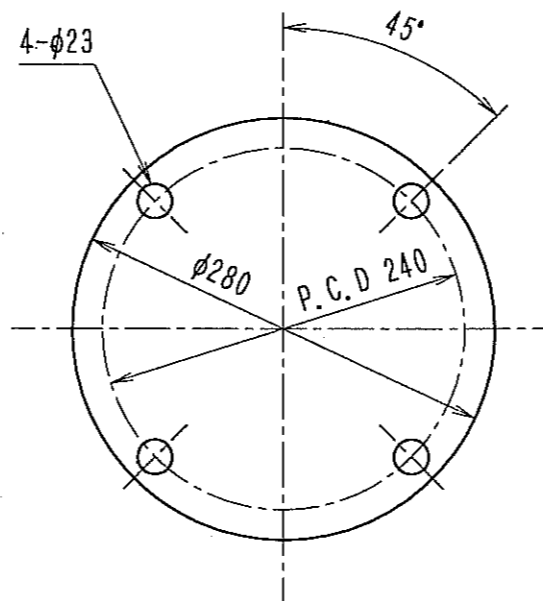
JIS 10K 150Aに準用 取付座詳細
