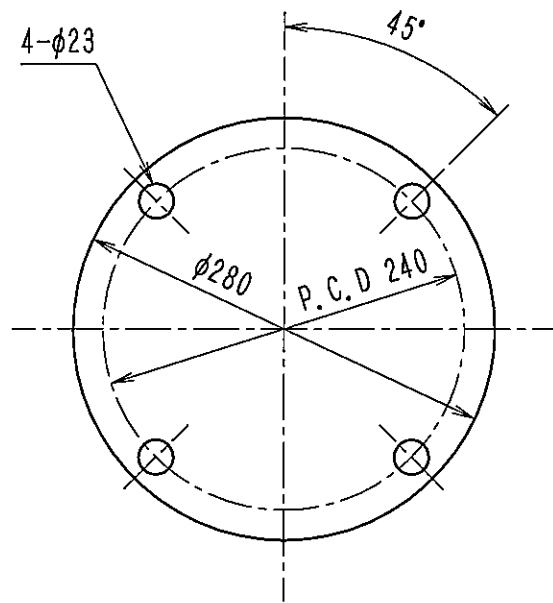
JIS 10K 150Aに準用 取付座詳細
