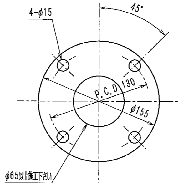
JIS 5K 65A 取付座詳細
