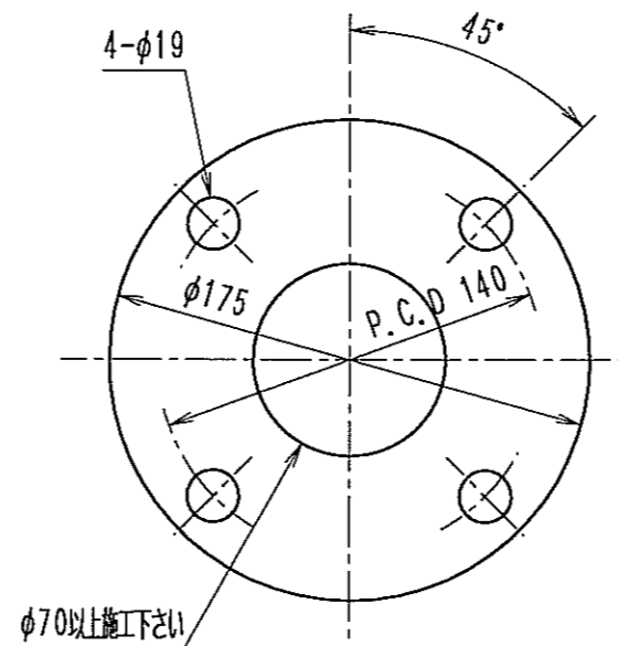
JIS 10K 65A 取付座詳細
